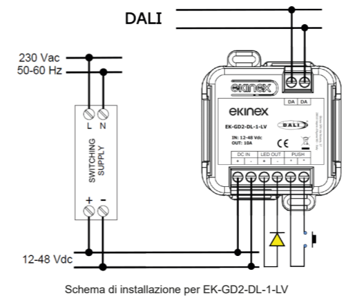
Schema di installazione per EK-GD2-DL-1-LV
