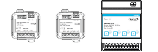
EK-GD2-DL-1-LV EK-GD2-DL-2-LV EK-GD1-DL-4-LV
