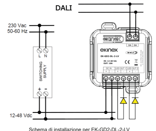
Schema di installazione per EK-GD2-DL-2-LV
