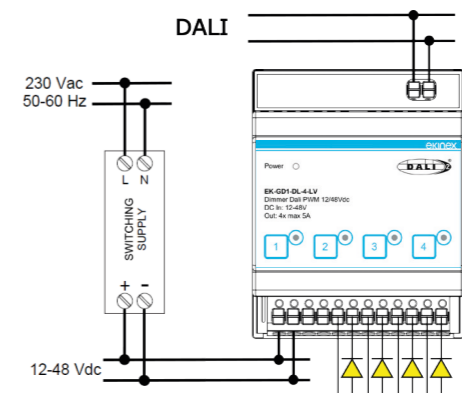
Schema di installazione per EK-GD1-DL-4-LV
